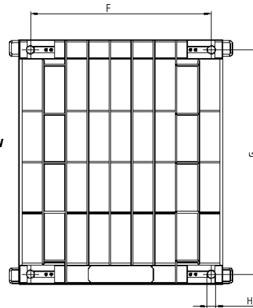
PUA574/579 dimensions
